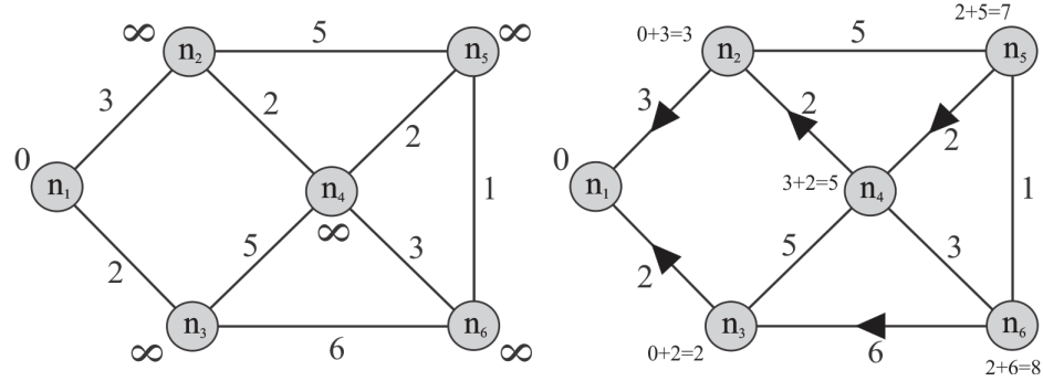
Figura 1.2: Algoritmo Dijkstra
